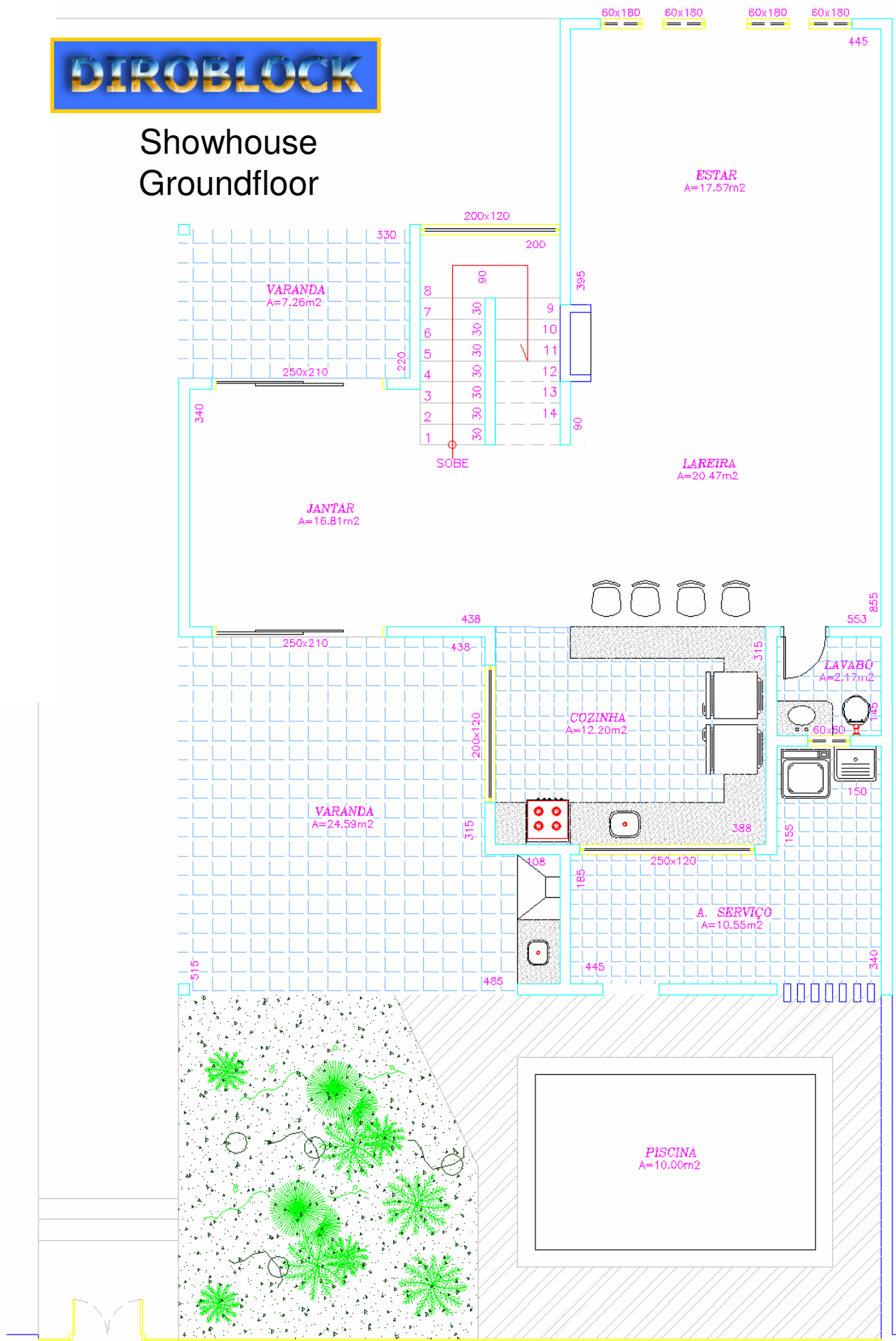
PLANTA PAV TÉRREO ESCALA 1/75
